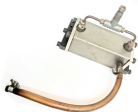
Cod.: 1335 Descrição: PNEUMATICO DA PINÇA DE ENTRADA GTO
